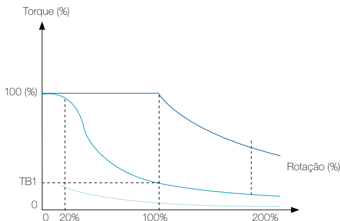
Gráfico torque x rotação típico para motor de 10 cv acionado por inversor CFW700
